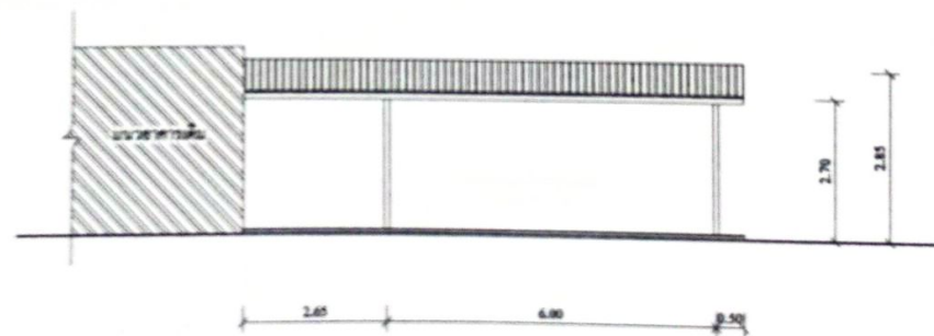
รูปด้านหลัง C SCALE 1:100
